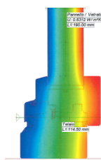
Isoterme - Vetro 48mm
